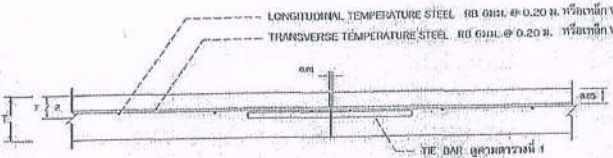
ขยายตัว LONGITUDINAL JOINT
