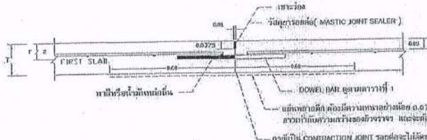
ขยายตัว RB CONSTRUCTION JOINT และ CONTRACTION JOINT
