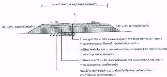
รูปตัดตามขวางถนนลูกรัง
