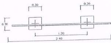
รูปแปลน 1:25
